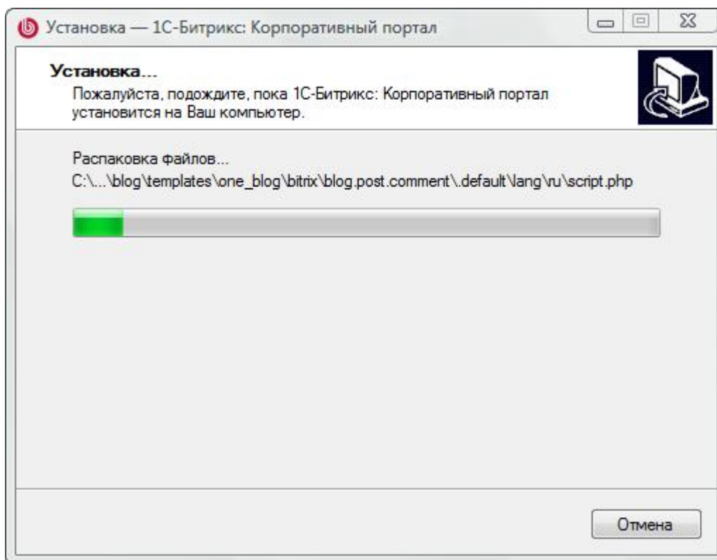
Рис. 2.8 Установка продукта
