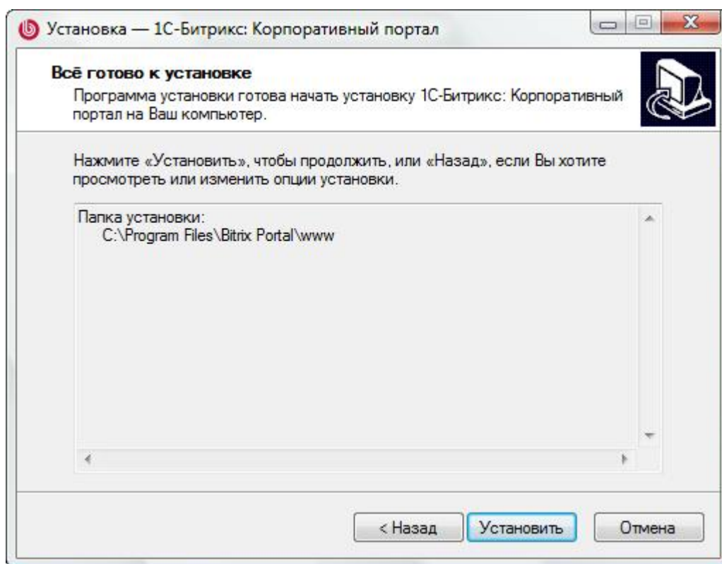
Рис. 2.6 Подтверждение установки
