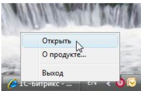
Рис. 2.11 Меню управления
