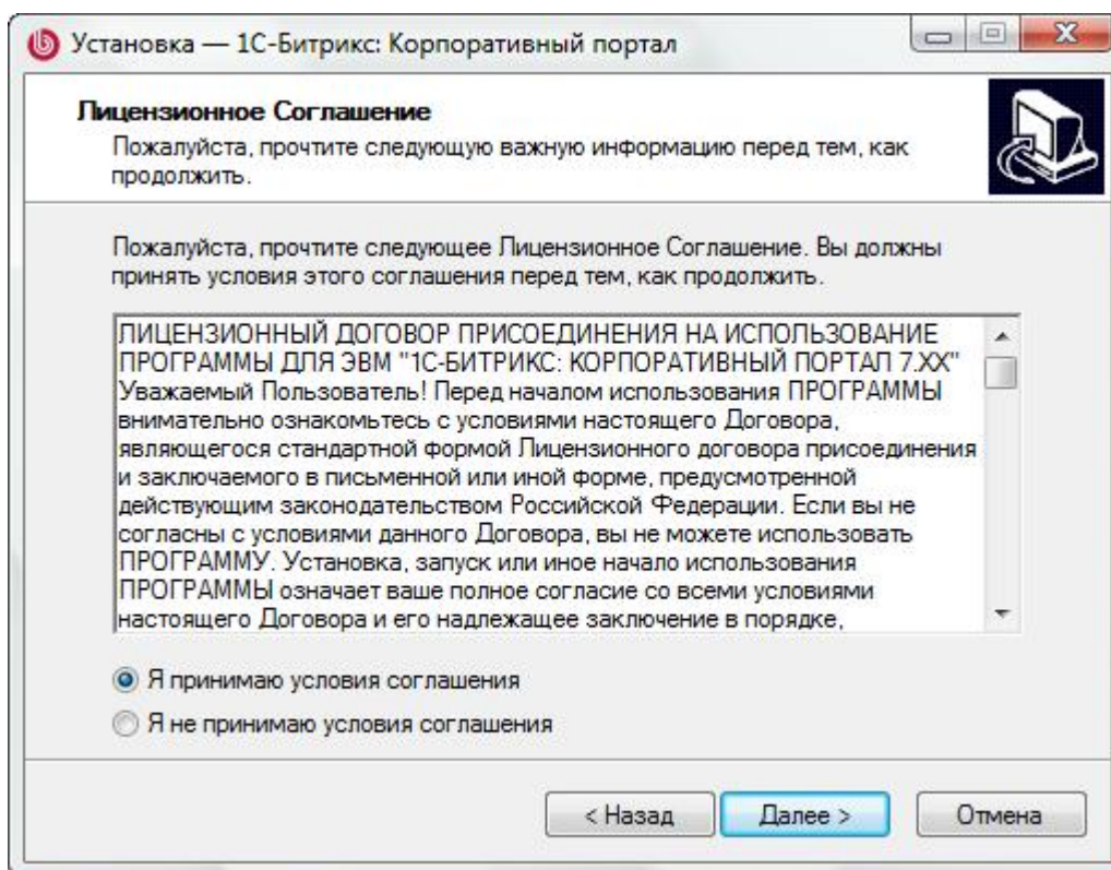
Рис. 2.2 Лицензионное соглашение
