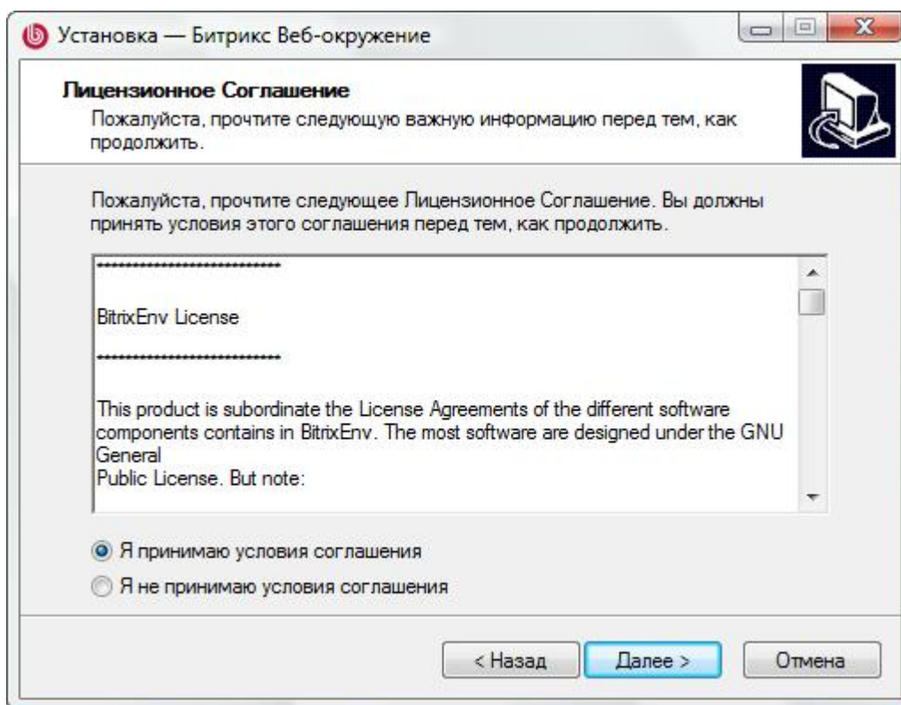
Рис. 3.3 Лицензионное соглашение
