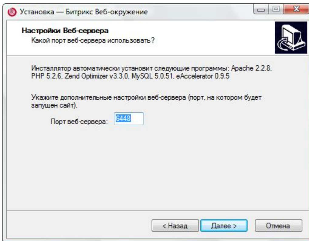
Рис. 3.7 Настройки Веб-сервера
