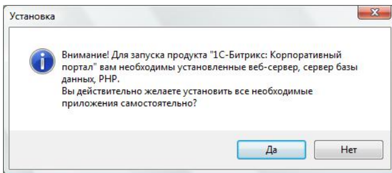
Рис. 2.4 Предупреждение
